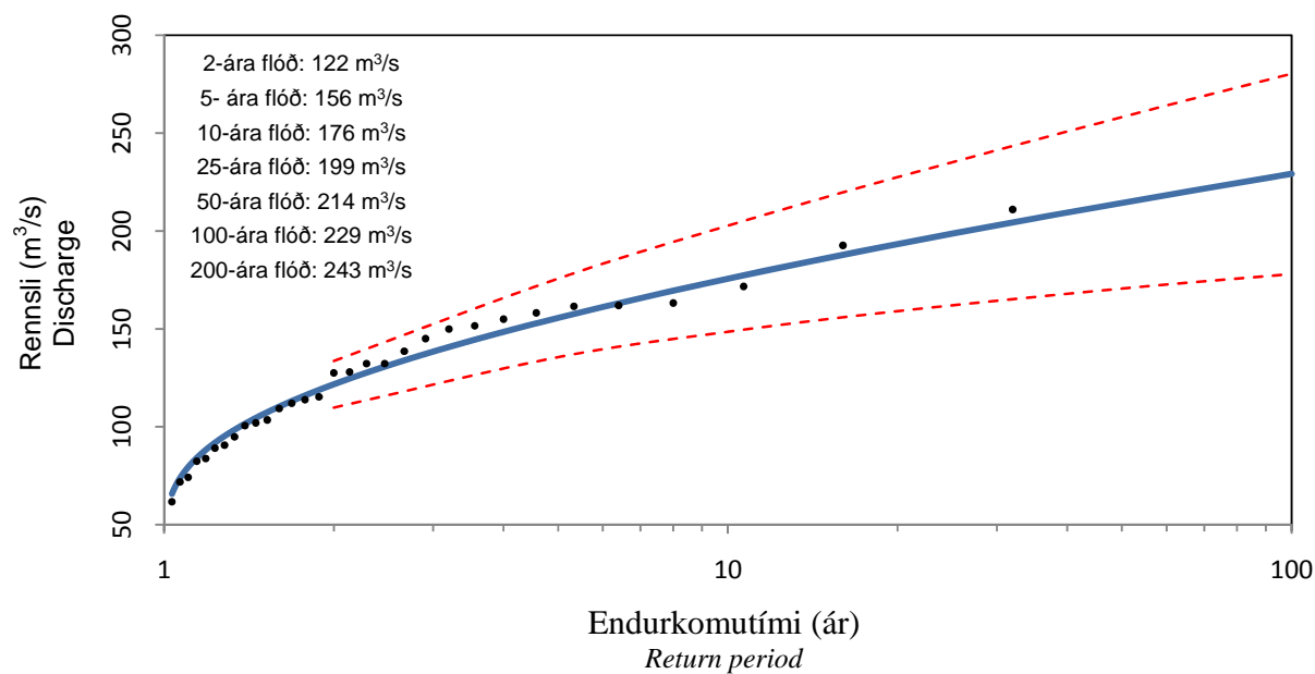
Reiknuð og mæld hæstu flóð áráanna 1977-2007 Calculated and measured maximum floods
