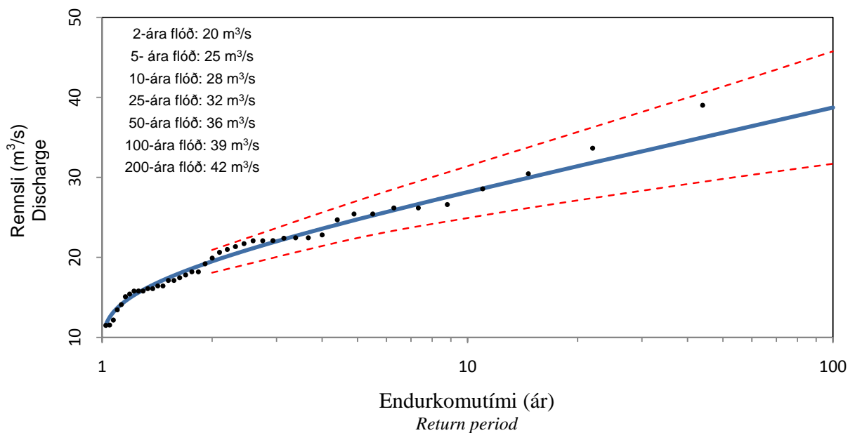
Reiknuð og mæld hæstu flóð árána 1965-2007 Calculated and measured maximum floods
