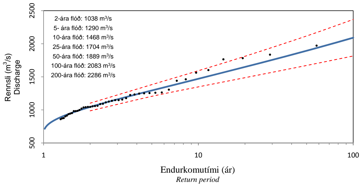
Reiknuð og mæld hæstu flóð árána 1951-2007 Calculated and measured maximum floods
