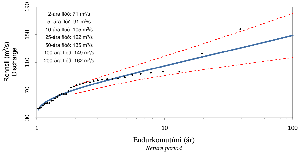
Reiknuð og mæld hæstu flóð árána 1970-2007 Calculated and measured maximum floods
