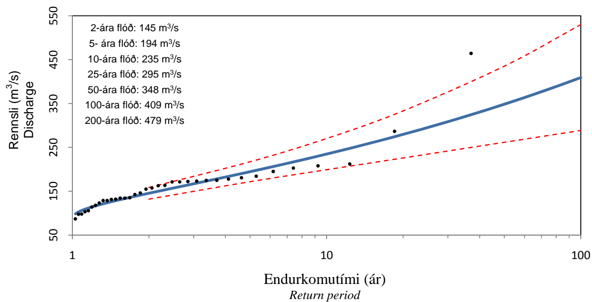
Reiknuð og mæld hæstu flóð árána 1972-2007 Calculated and measured maximum floods
