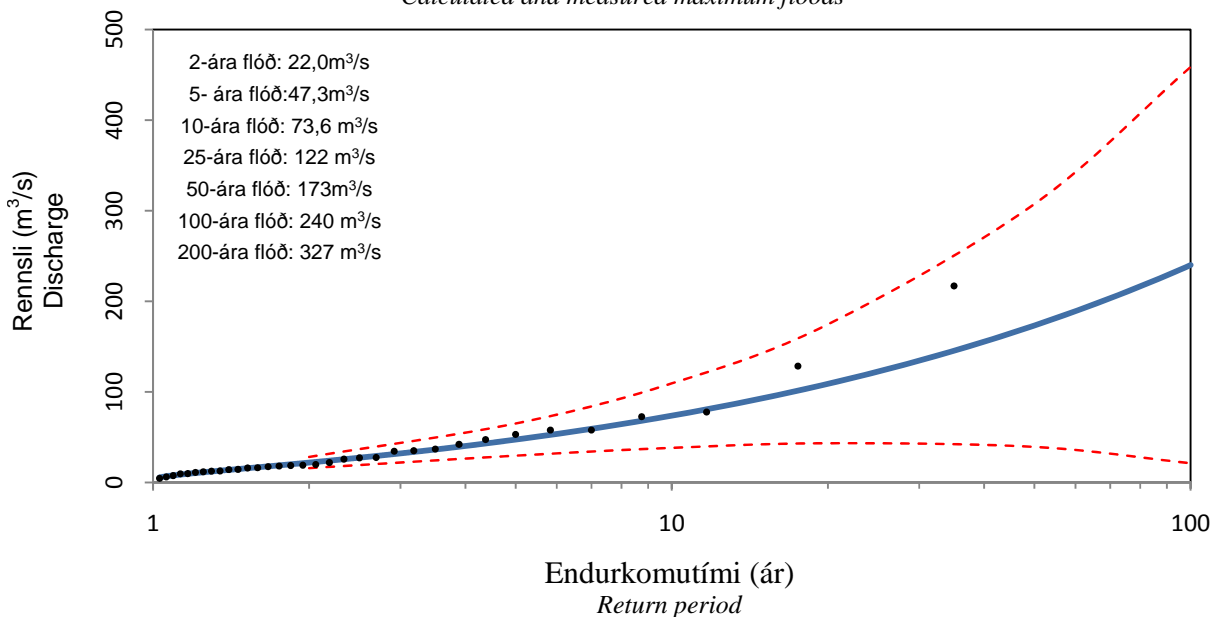
Reiknuð og mæld hæstu flóð árána 1974-2007 Calculated and measured maximum floods
